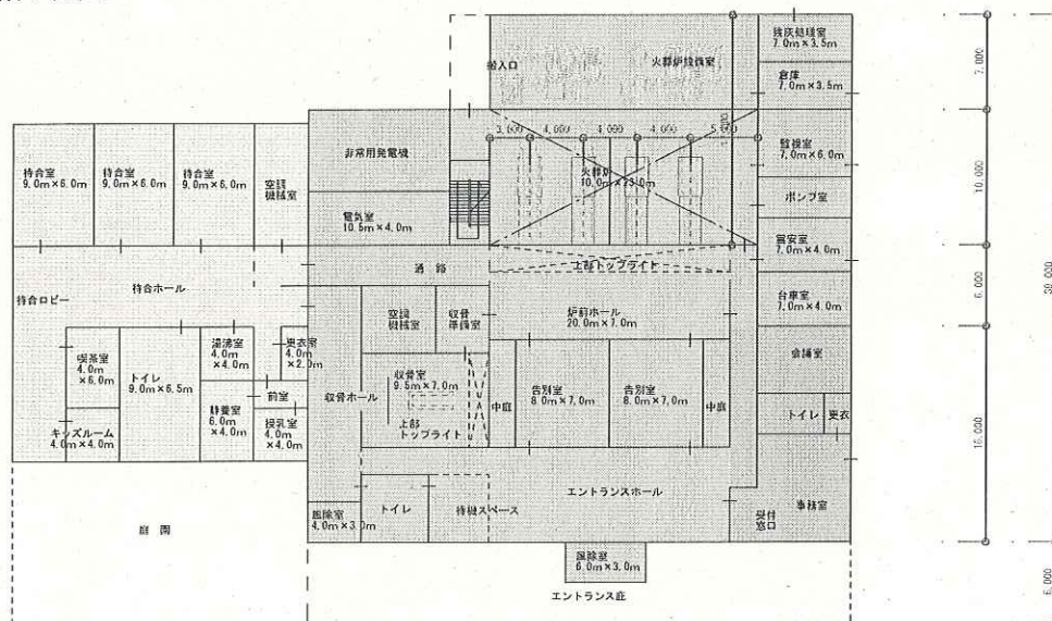
1 階平面図
