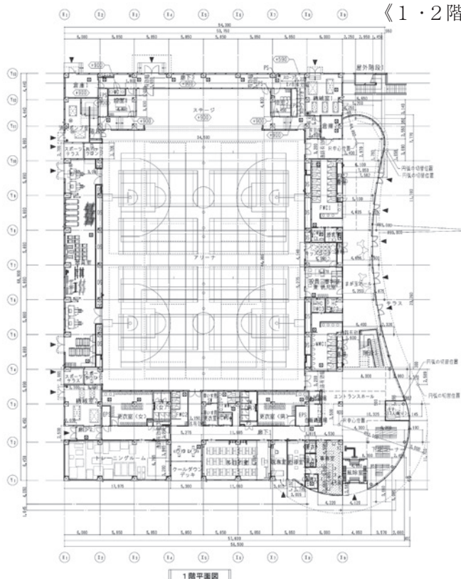
《1・2階平面図》
