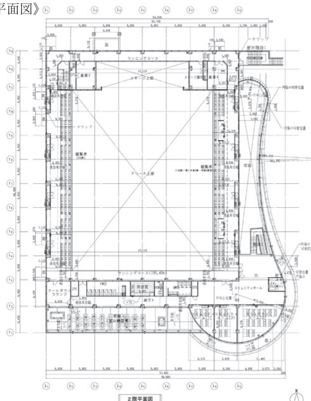
《1・2階平面図》
